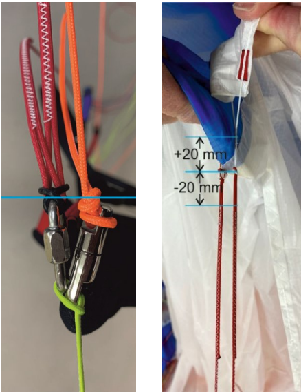
Fig. 12 Meßpunkte für Bremsleinen Schnellcheck
