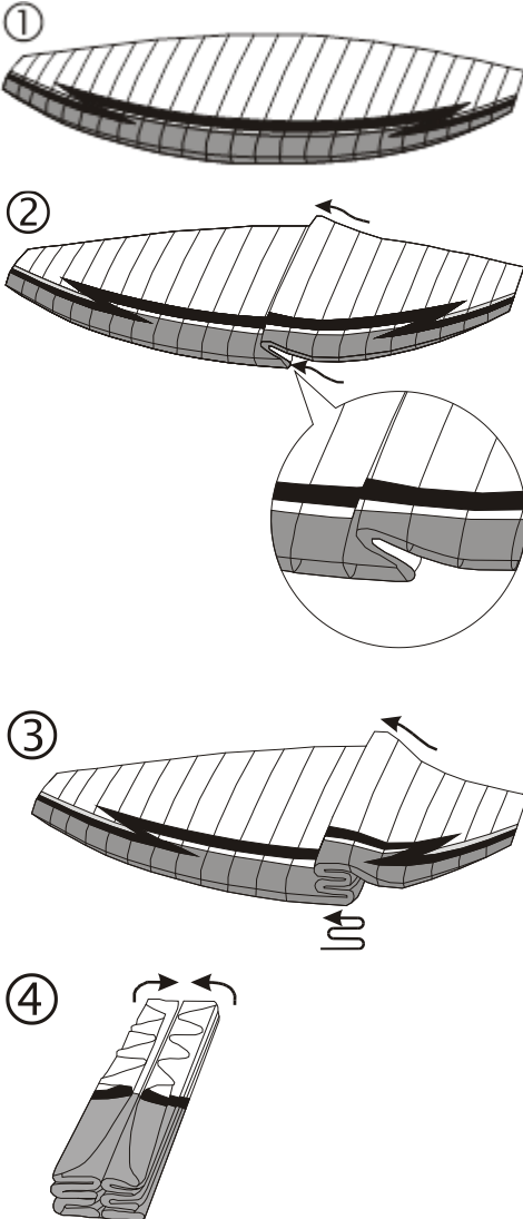
Fig. 11 Bildfolge Zusammenlegen des MIURA 2 RS
