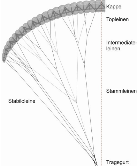
Fig. 1 Gittermodell MIURA 2 RS
