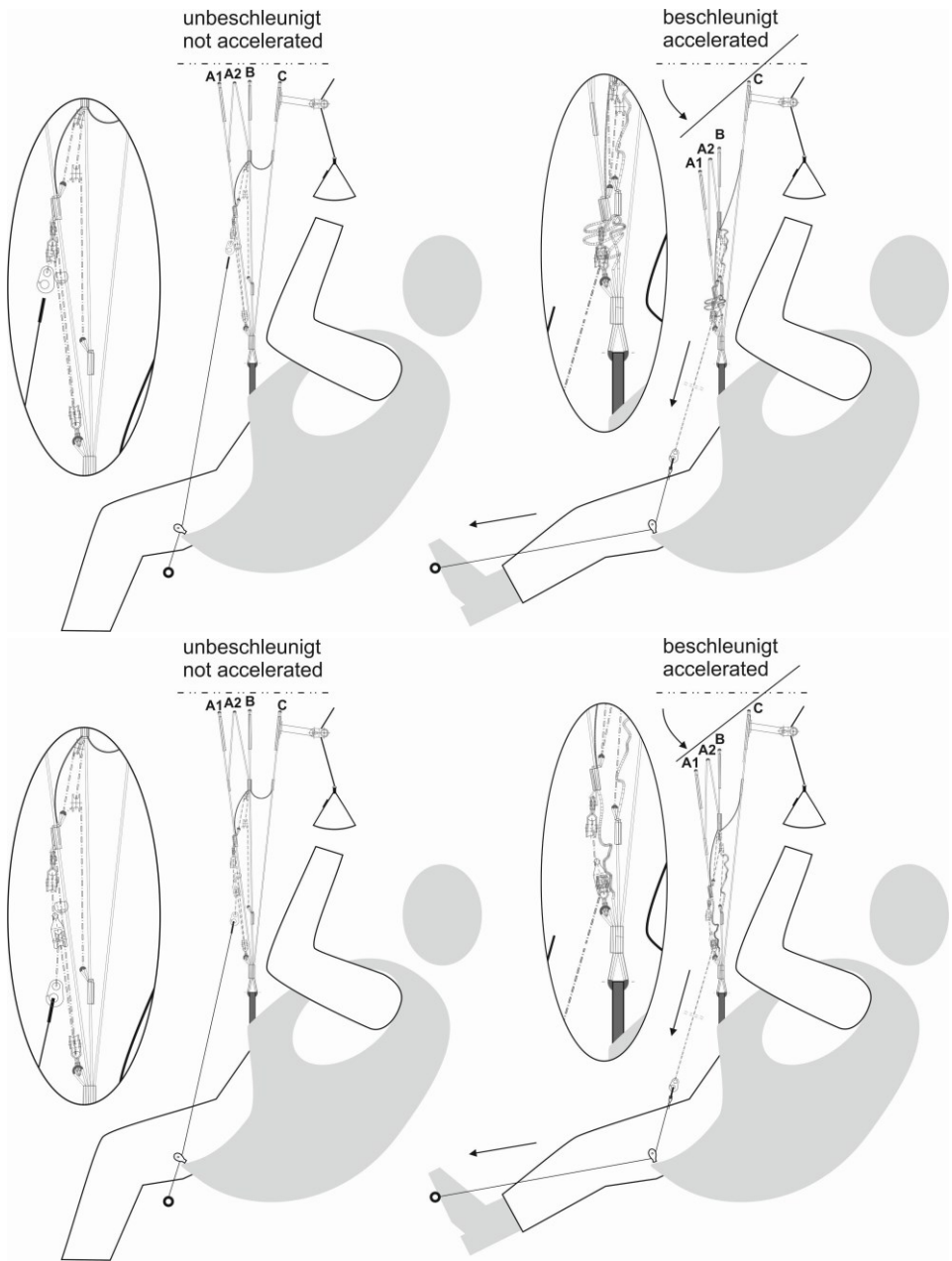
Fig. 6 Funktionsweise Fußbeschleuniger MIURA 2 RS ohne (obere Abbildung) und mit Speedlimiter (untere Abbildung)
